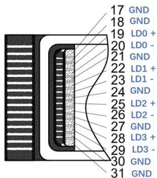
TOSA脚位定义
